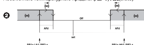
Абсолютные температурные пределы ( Att=0 ) Abs(olute)
